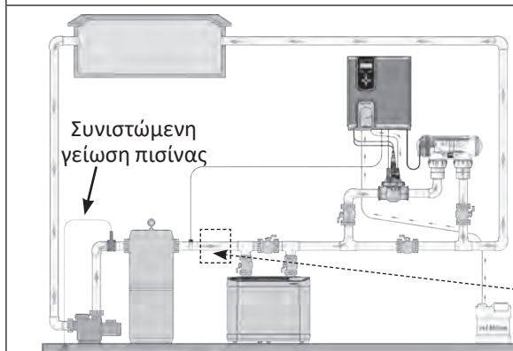
Εγκατάσταση με σύστημα θέρμανσης
