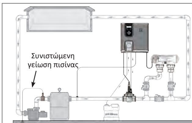
Εγκατάσταση σε σειρά
